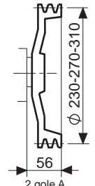
Puleggia Pulley Polea Poulie Keilriemenscheibe
